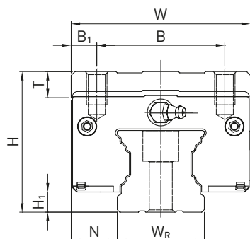
Rozměry vozíků CG
